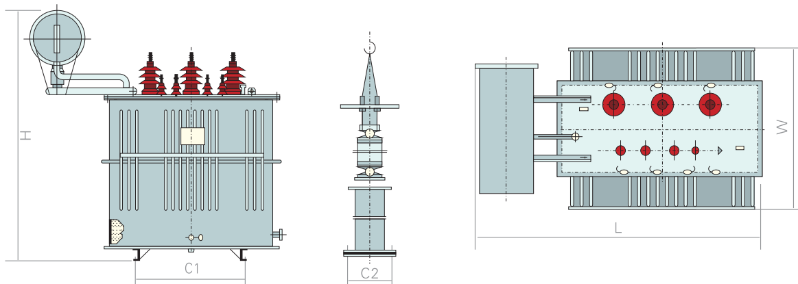
S9-50~1600/35变压器
